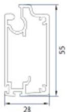
H95 28 x 55mm Förstärkt underlist med plats för dubbla tyngder. Dubbla tyngder krävs för vissa storlekar
