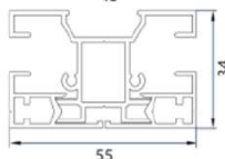
H98 55 x 34mm Dubbelgejder för delning i hel kassett. Används tillsammans med H96 Tredelad med dold infästning. Skruvas ihop vid montering.
