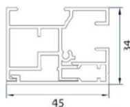
H96 45 x 34mm Tvådelad med dold infästning Skrivas ihop vid montering
